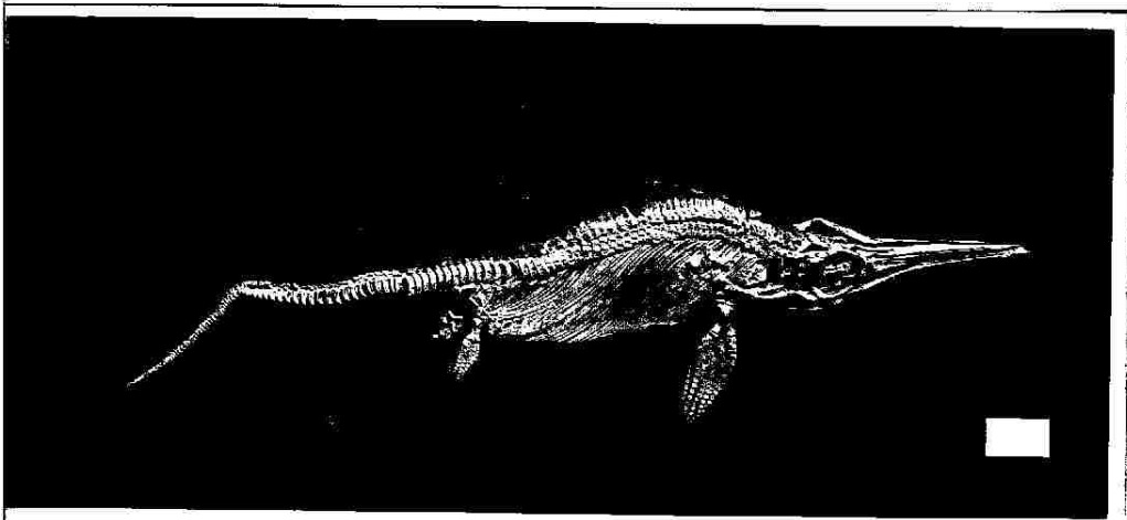
Ichthyosaurus quadriscissus Qu. (emend. E. Fraas) mit vollständiger Hautbekleidung, 2 m lang, oberer Lias Holzmaden.
